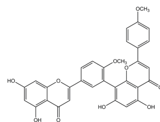
Isoginkgetin, (product # 83513)
